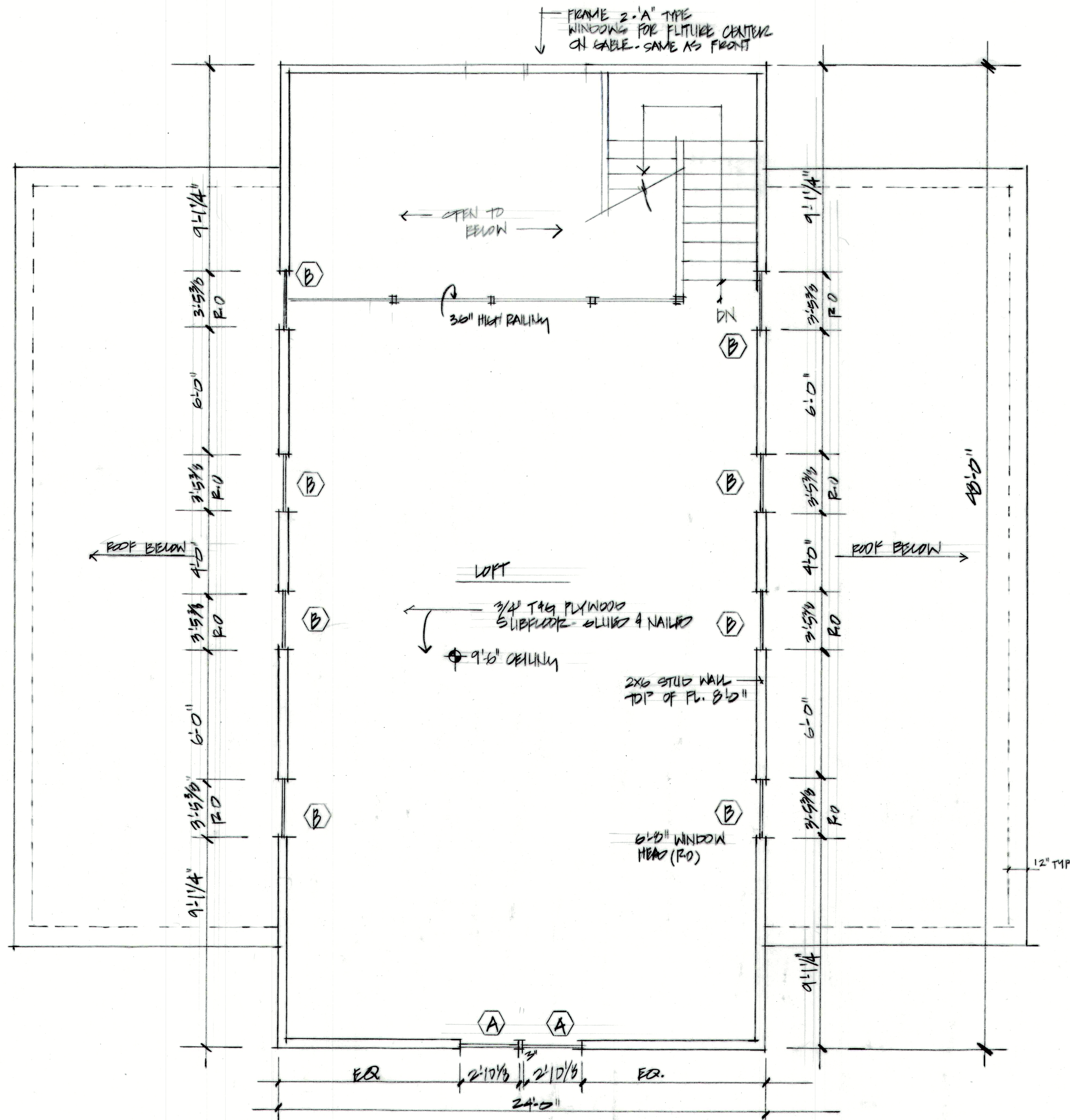
LOFT PLAN
